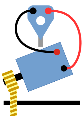
Suivant la manière que l'on positionne le moteur, cage ouverte vers le bas ou le haut
