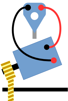
Suivant la manière que l'on positionne le moteur, cage ouverte vers le bas ou le haut
